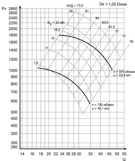
Рис. 12б - Дк=1,05 Дном
