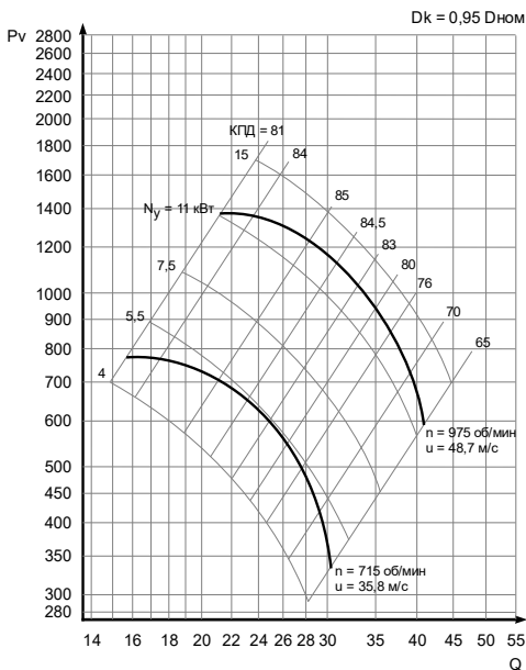
Рис. 12а - Дк=0,95 Дном
