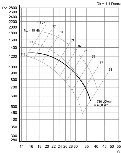
Рис. 12в - Дк=1,1 Дном
