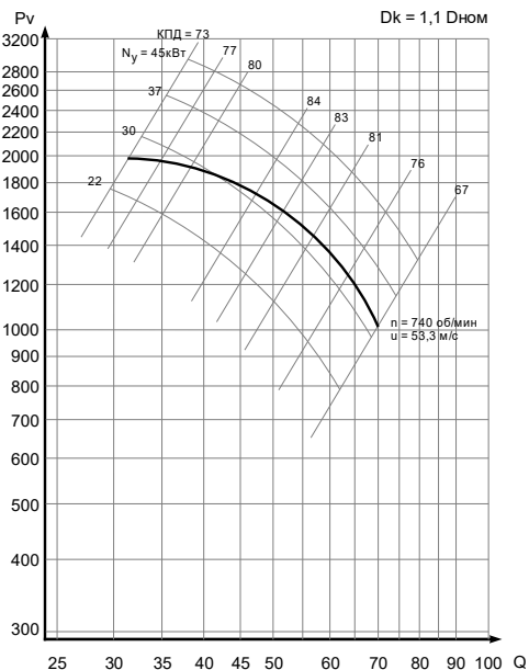
Рис. 13г - D_k=1,1 \text{ Дном}
