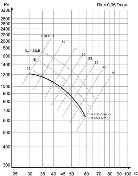
Рис. 13б - D_k=0,95 \text{ Дном}
