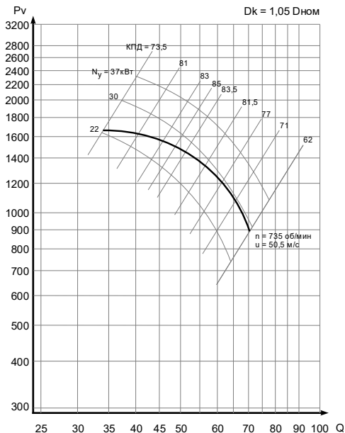
Рис. 13в - D_k=1,05 \text{ Дном}
