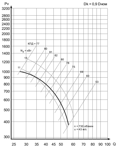
Рис. 13а - D_k=0,9 \text{ Дном}
