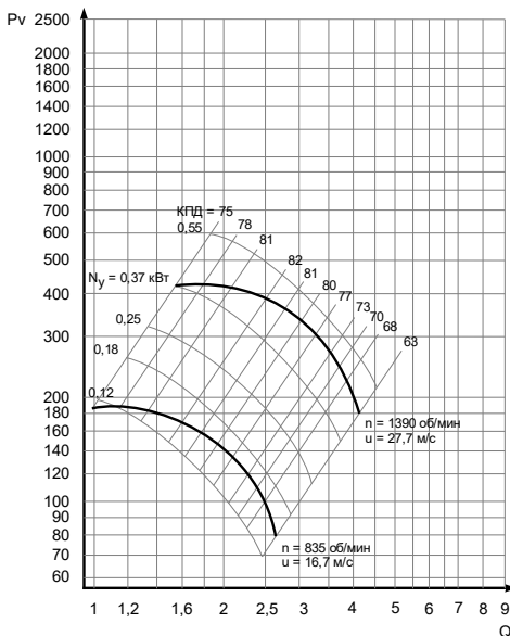
Рис. 8б - D_k=0,95 D_{ном}
