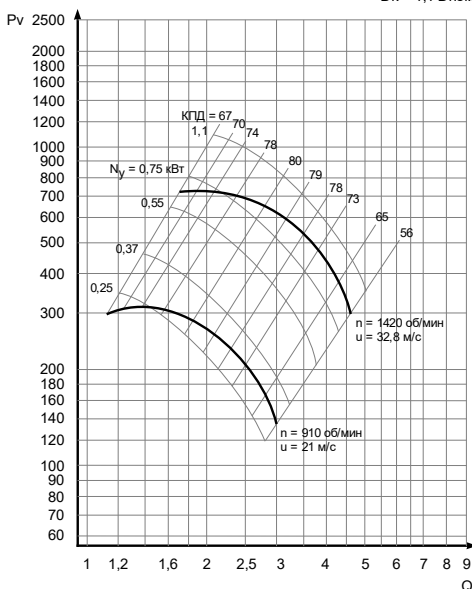
Рис. 8г - D_k=1,1 D_{ном}
