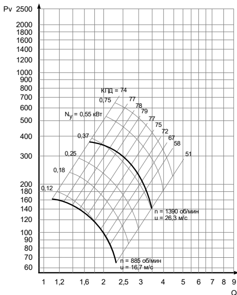
Рис. 8а - D_k=0,9 D_{ном}
