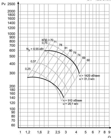
Рис. 8в - D_k=1,05 D_{ном}
