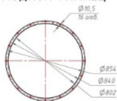
ВЫХОДНОЙ ФЛАНЕЦ
