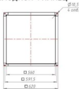
ВЫХОДНОЙ ФЛАНЕЦ
