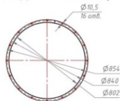
ВЫХОДНОЙ ФЛАНЕЦ
