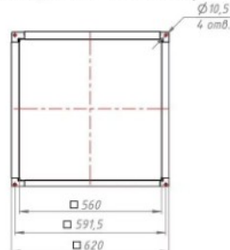
ВЫХОДНОЙ ФЛАНЕЦ
