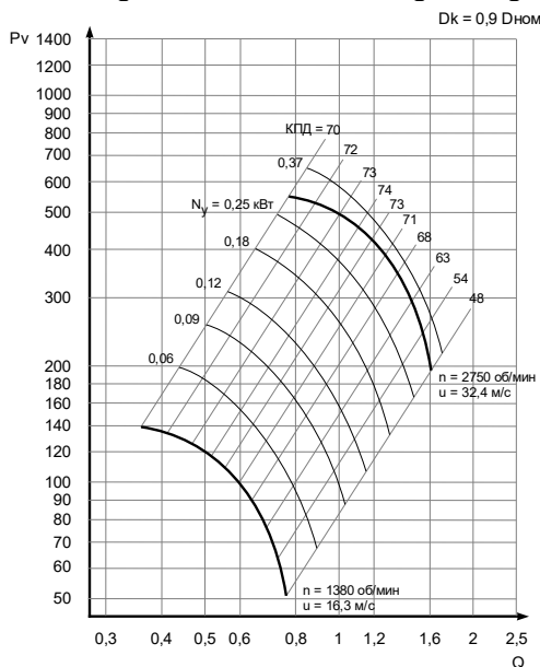
Рис. 6а - Dk=0,9 Дном
