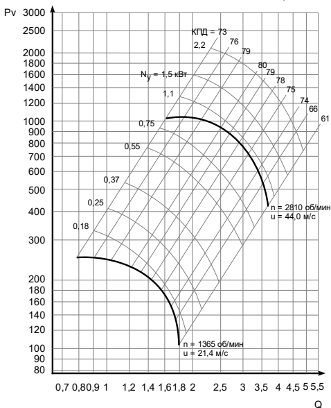
Рис. 7б - D_k=0,95 D_{ном}
