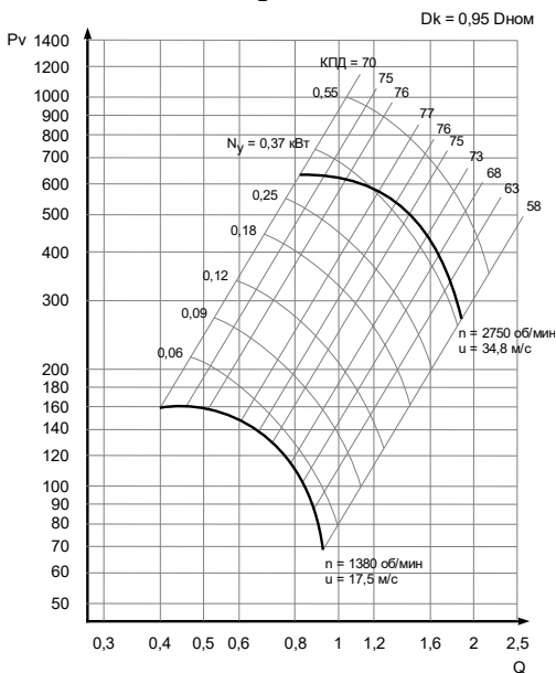
Рис. 6б - Dk=0,95 Дном
