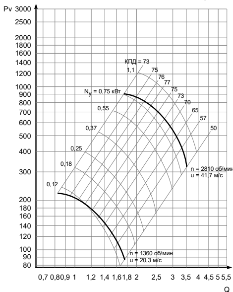
Рис. 7а - D_k=0,9 D_{ном}
