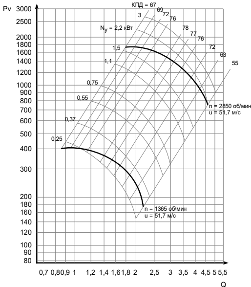
Рис. 7г - D_k=1,1 D_{ном}
