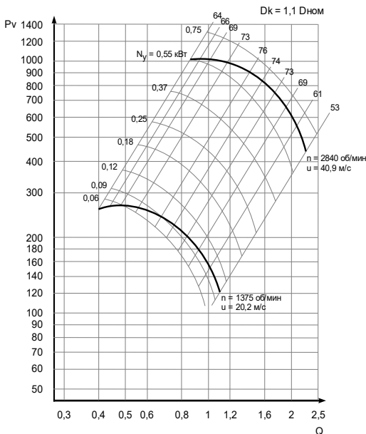
Рис. 6г - Dk=1,1 Дном
