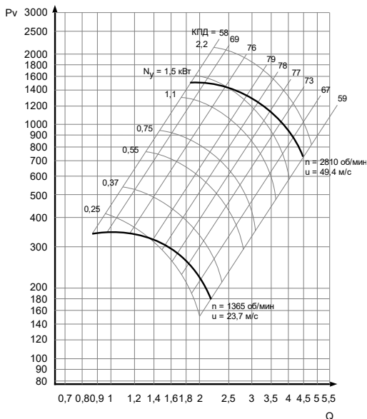
Рис. 7в - D_k=1,05 D_{ном}
